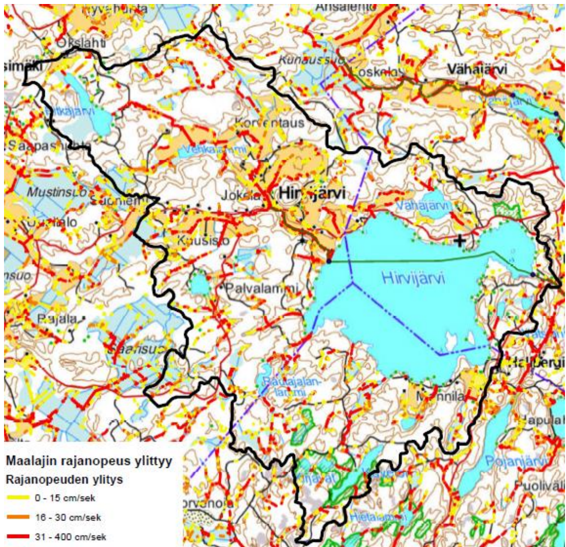
Kuva 12. Uoma-analyysin avulla voidaan kuvata ojaston eroosioriskiä eli ylittääkö veden virtausnopeus ojassa maalajin rajanopeuden. Punaisella kuvatuissa ojissa eroosioriski on suurin, oranssilla kuvatuissa riski on keskimääräinen ja keltaisella kuvatuissa riski on vähäisin.
