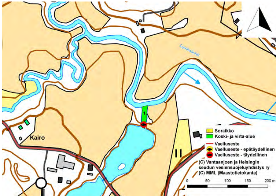
Kuva 43. Lepsämänjokeen laskevan Lakistonjoen Kairon (1) virta-alue.
