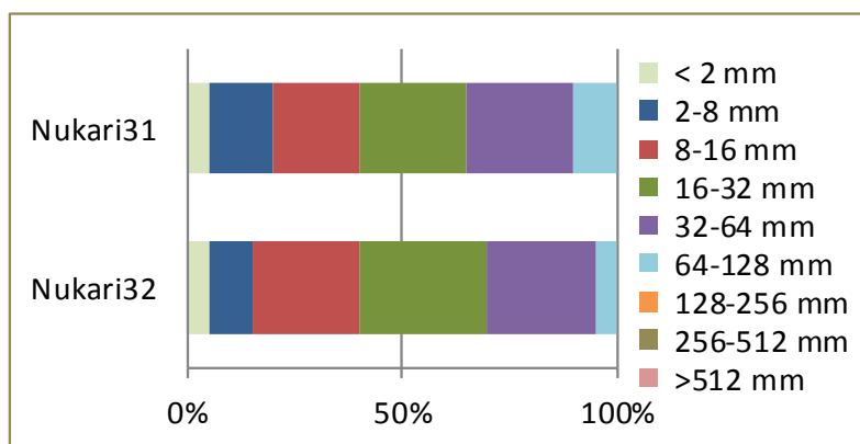
Kuva 35. Nukarin koskien Harrikosken alapuolen inventoitujen soraikkojen raekokojen prosentuaaliset osuudet.
