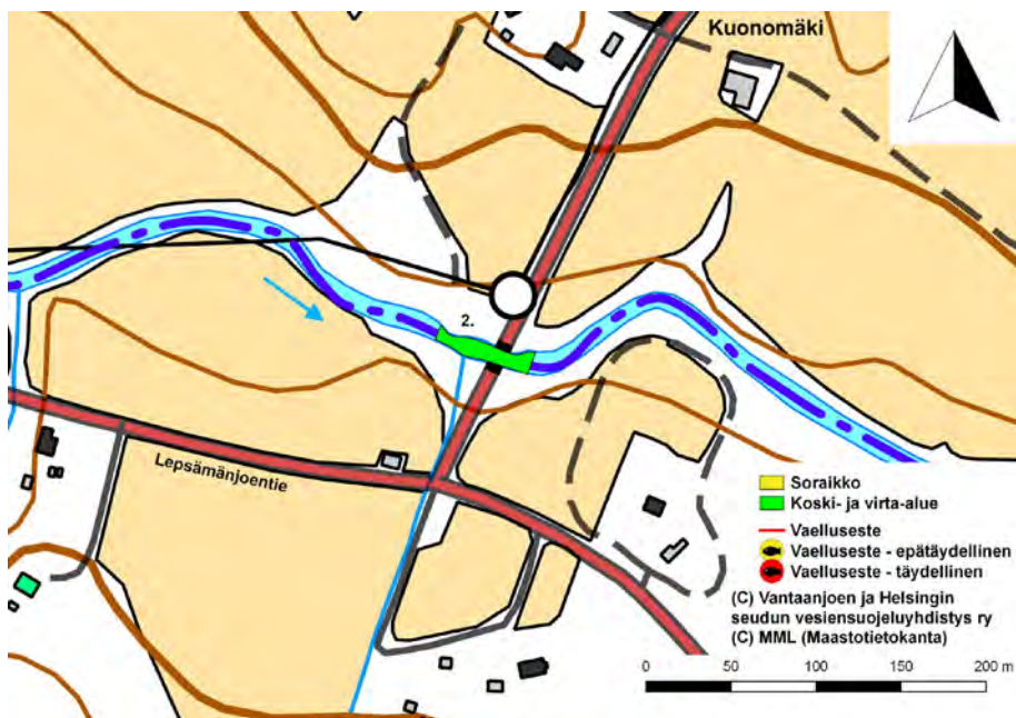
Kuva 44. Lepsämänjoen Kuonomäen (2) virta-alue.
