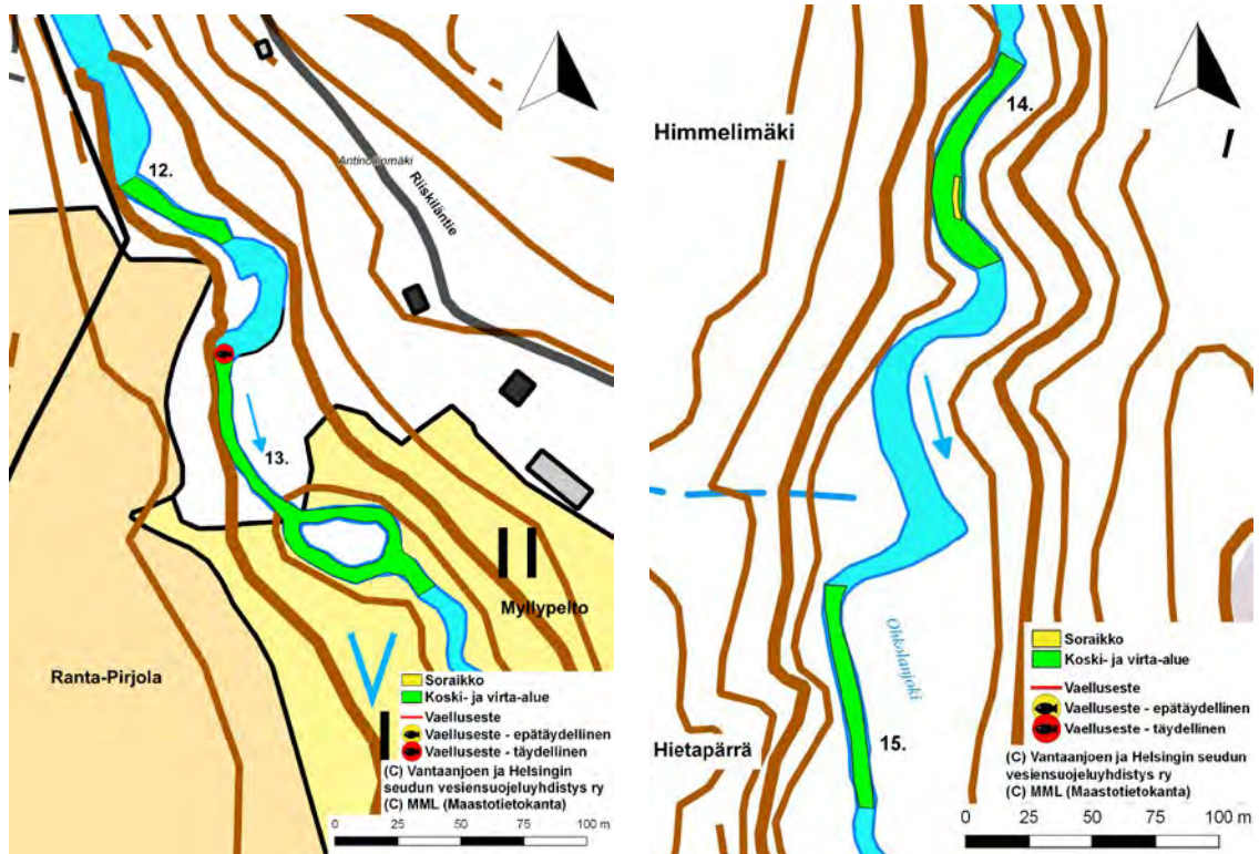
Kuvat 65 & 66. Ohkolanjoelta määritetyt koski- ja virta-alueet 12–13 (vasen kuva: karttakuva 6) ja 14–15 (oikea kuva: karttakuva 7).
