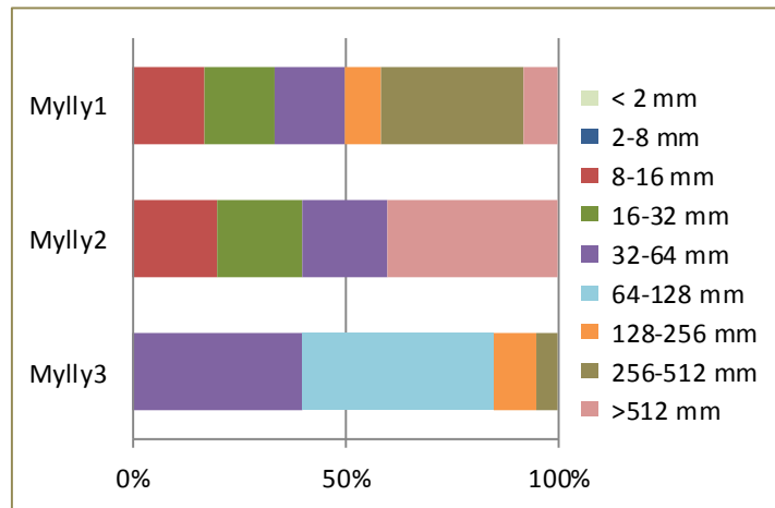
Kuva 13. Myllykosken inventoitujen soraikkojen raekokojen prosentuaaliset osuudet.
