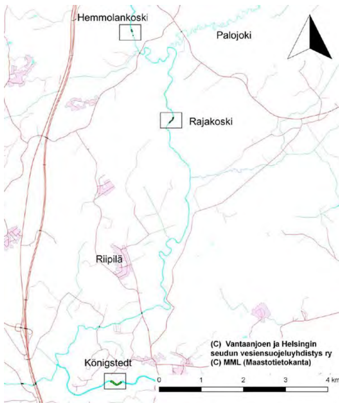
Kuva 4. Vantaanjoen pääuoman alaosiensien vuonna 2017 kartoitetut koski- ja virta-alueet.
