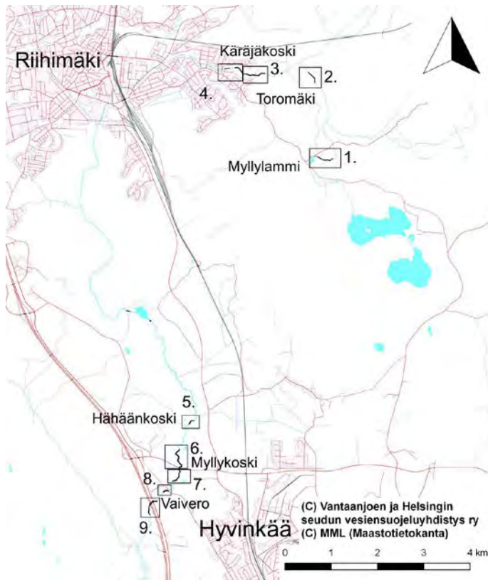
Kuva 2. Myllylammin ja Vaiveron väliseltä alueelta vuonna 2017 määritetyt koski- ja virta-alueet.
