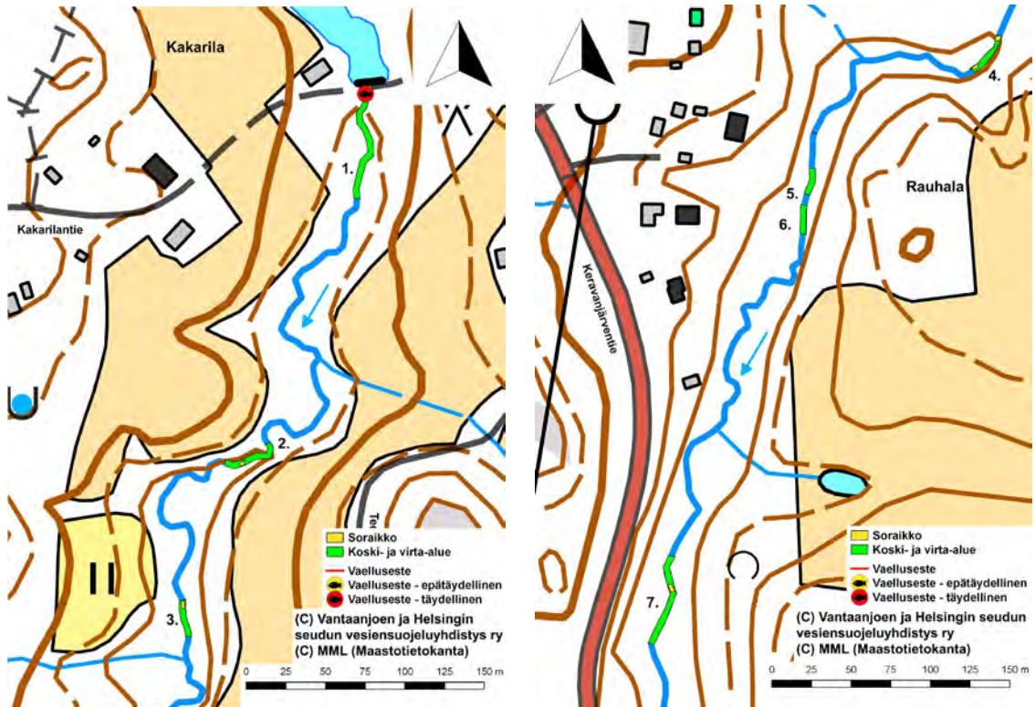
Kuvat 57 & 58. Ohkolanjoelta määritetyt koski- ja virta-alueet 1–3 (vasen kuva: karttakuva 1) ja 4–7 (oikea kuva: karttakuva 2).
