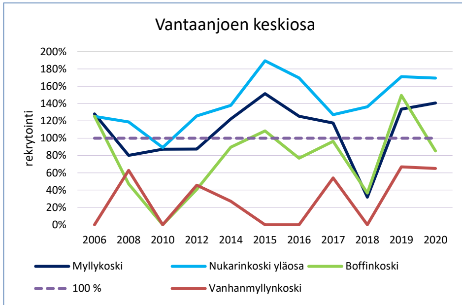
Kuva 13. Vantaanjoen keskiosan koealojen rekrytointistatus vuosina 2006–2020.
