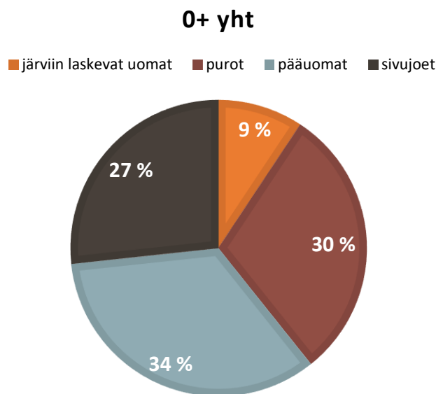
Kuva 4. Vantaanjoen vesistöalueen taimenen poikastuotantopotentiaalin jakautuminen eri uomatyyppeihin välillä.
