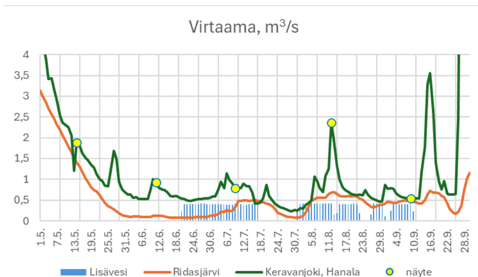
Kuva 6.6. Keravanjoen vuorokausikeskivirtaama (m 3 /s) Hanalassa ja jokeen johdetun lisäveden virtaama ja Ridasjärven lähtövirtaama kesällä 2024. (tiedot: SYKE/Avoin tieto ja KUVES)
