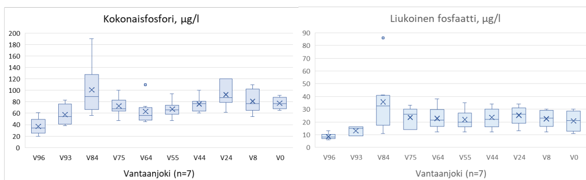
Kuva 3.4. Kokonaisfosforin ja liukkeen fosfaatin pitoisuudet Vantaanjoessa (7 näytettä/havaintopaikka) vuonna 2024. Kuvassa ruudun alareuna vastaa alaneljännestä ja yläreuna yläneljännestä, ruudun sisään piirretty viiva vastaa mediaania ja rasti keskiarvoa. Janojen päät ovat ääriarvoja. Havainnoissa on poikkeavia arvoja eli yli 1,5 laatikon korkeuden päässä laatikon reunasta, jotka on esitetty janan ulkopuolisina pisteinä.
