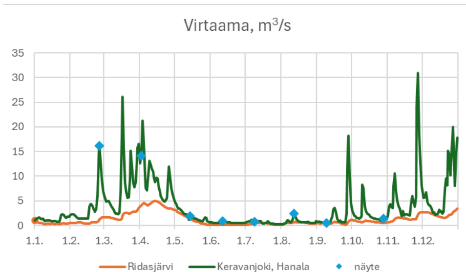
Kuva 6.1. Ridasjärvestä lähtevän veden virtaama ja Keravanjoen virtaama (m³/s) Hanalassa vuonna 2024 sekä näytekerrat joen perusseurantapaikoilla. (tiedot: SYKE/Avoin tieto)
