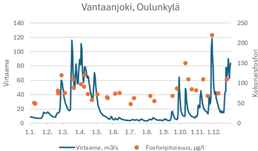
Kuva 2.4. Vantaanjoen vuorokausikeskivirtaama (m³/s) Helsingin Oulunkylässä vuonna 2024 sekä kokonaisfosforipitoisuus Vantaanjoen alajuoksulla. (tiedot: SYKE/Avoin tieto 24.1.2025)
