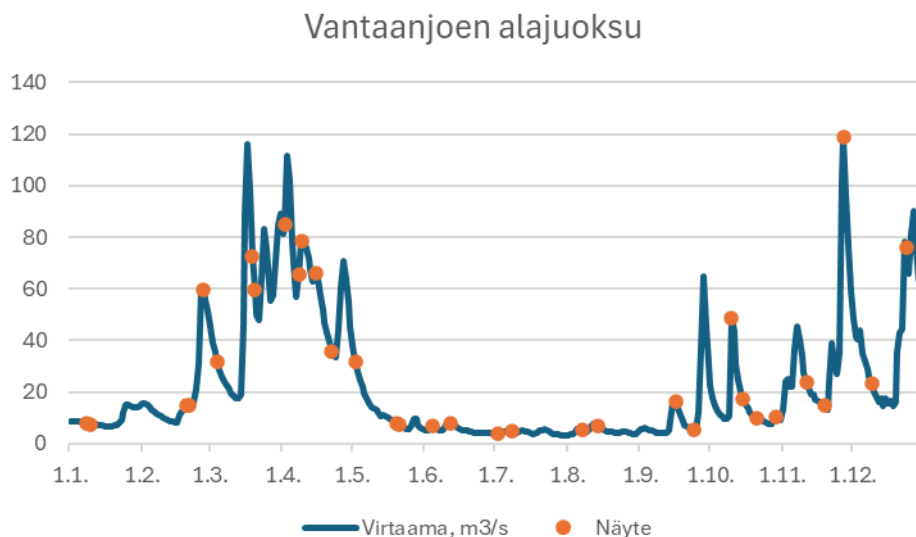
Kuva 10.1. Vantaanjoen vuorokausikeskivirtaama Oulunkylässä (m³/s) ja joen alajuoksulta (Vantaa 4,2 ja Vantaa 1,3) otettujen näytteiden ottoajankohdat vuonna 2024.
