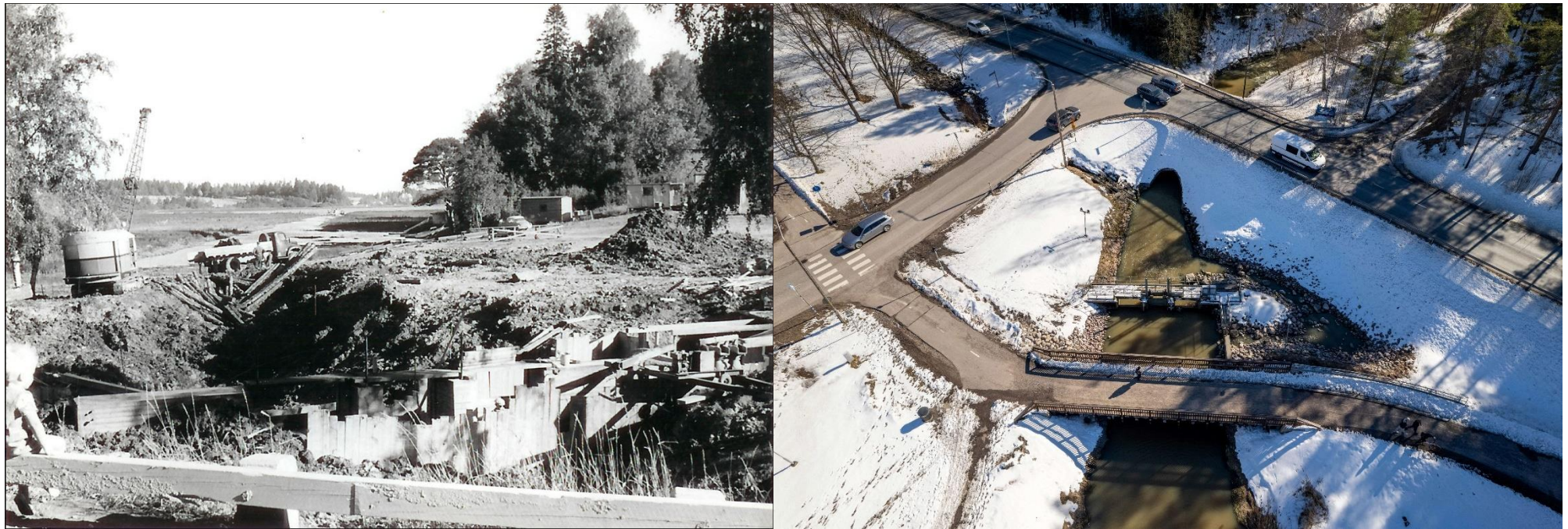
Kuva 4. Tuusulanjärven luusuaan rakennettu säännöstelypato rakennusvaiheessa vuonna 1958 (vas.) ja säännöstelypato kalateineen maaliskuussa vuonna 2023 (oik.). Kuvat: Koskensillan padon rakennus 1958, kuvaaja Vesa Savimaa; Tuusulanjärven pato ja kalatie, VHVSY kuva-arkisto.
