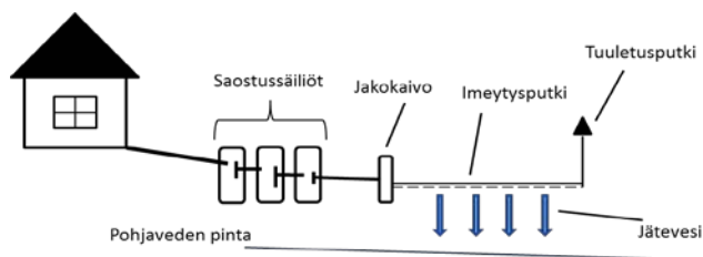
Kuva 1. Maahanimeyttämön periaate.
