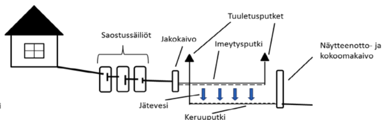
Kuva 2. Maasuodattamon periaate.
