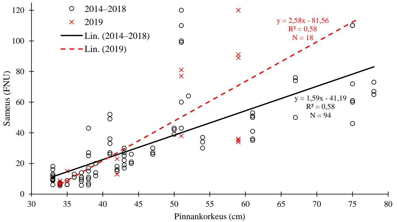
Kuva 21. Luhtajoen sameuden ja vedenkorkeuden suhde eri ajanjaksoina. Vuonna 2019 sameus oli keskimäärin suurempaa kuin aikaisempina vuosina. Tarkastelussa on käytetty näytepisteiden L37, L55 ja L57 sameustuloksia sekä Luhtajoen vedenkorkeuden anturin mittauksia.
