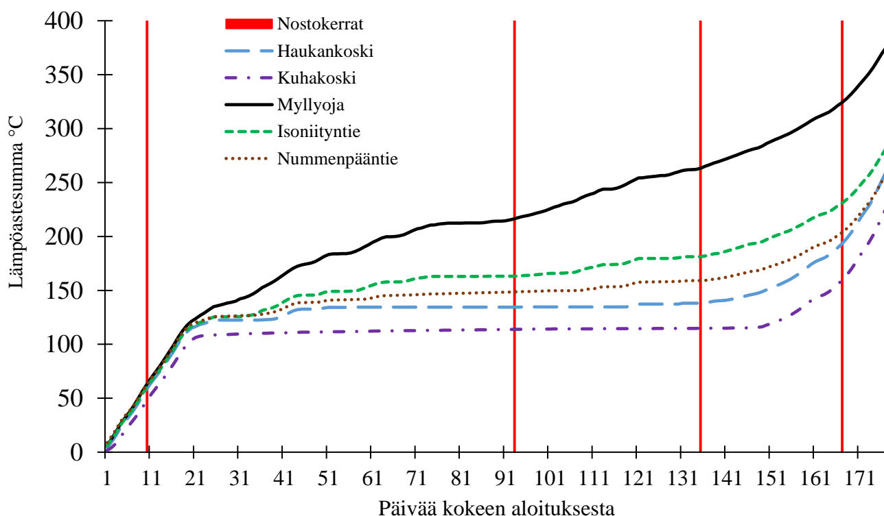
Kuva 20. Mädinhaudontakokeen päiväastekertymät eri tutkimusalueilla kokeen aloituksesta kokeen päättymiseen asti (31.10.2018–25.4.2019). Kuhakosken HOBO-mittari lähti korin mukana liikkeelle 10.4. eikä mitannut enää veden lämpötilaa, minkä takia viimeiset 15 päivää on arvioitu Haukankosken lämpötiloja vastaaviksi.
