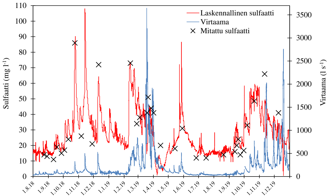
Kuva 23. Laskennalliset sulfaattipitoisuudet, virtaama ja mitatut sulfaattipitoisuudet Lepsämänjoen mittausasemalla hankkeen kalastotutkimusten aikana.
