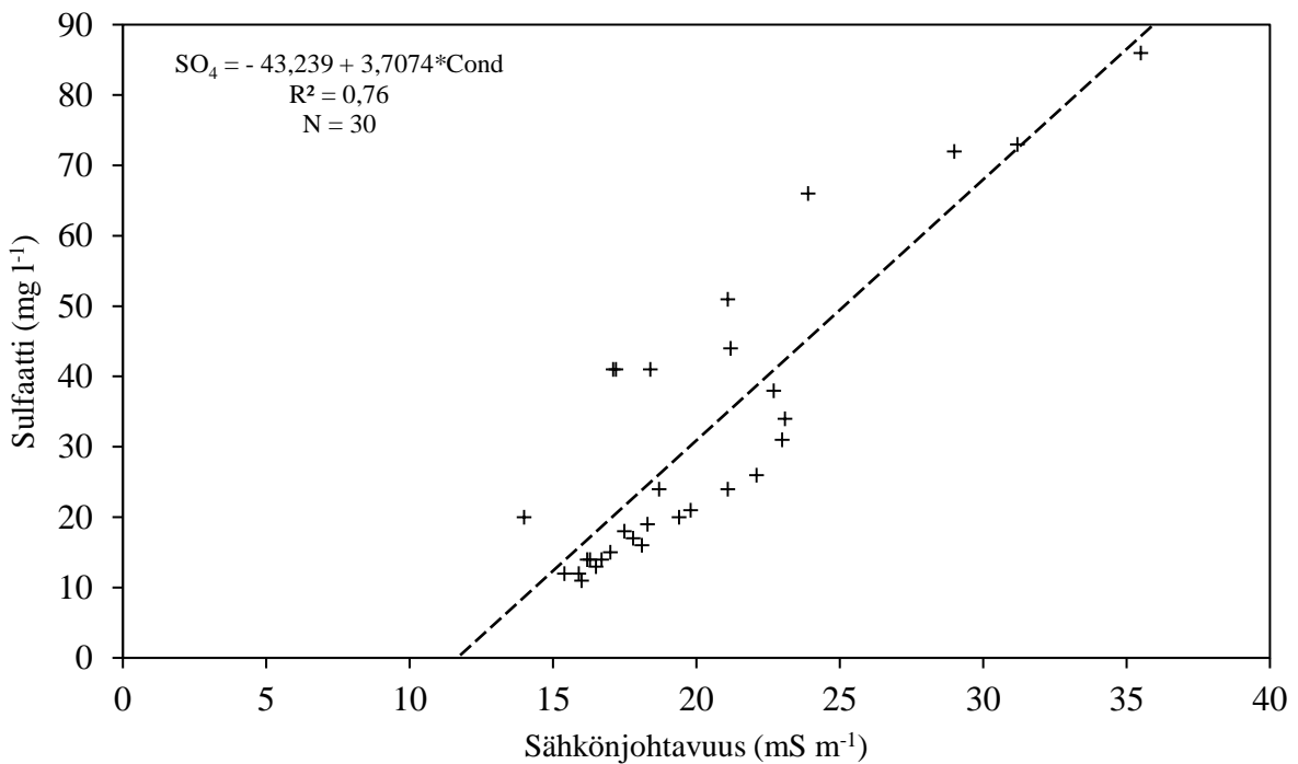
Kuva 22. Sulfaattiarvojen laskemiseen sähkönjohtavuudesta käytetty kaava määritettiin Lepsämänjoen vertailunäytteiden (näytteenottopiste Le50) avulla.
