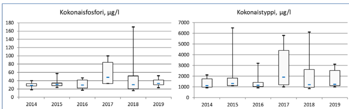
Kuva 4.4. Kokonaisravinteiden pitoisuudet Vantaanjoen Käräjäkoskessa vuosina 2014–2019. Kuvan laatikkokaaviossa laatikon alareuna vastaa alaneljännestä, yläreuna yläneljännestä, alin ja ylin poikkiviiva on aineiston pienin ja suurin arvo ja laatikossa oleva poikkiviiva on mediaani. Näytteitä havaintopaikalta on otettu 8 kpl/vuosi, paitsi 2017 10 kpl.
