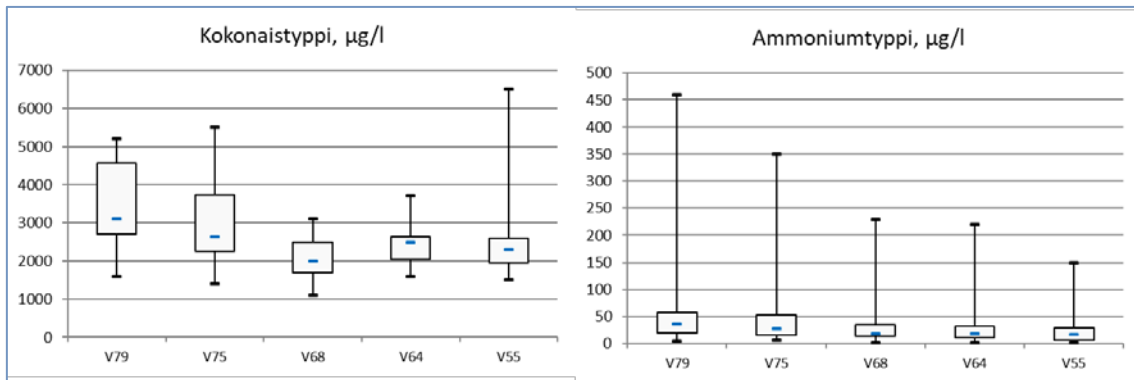
Kuva 4.29. Vantaanjoen typpipitoisuus Kaltevan puhdistamon ylä- (V75 ja V68) ja alapuolella (V64, V55) vuosina 2017–2019. Kuvan laatikkokaaviossa laatikon alareuna vastaa alaneljännestä, yläreuna yläneljännestä, alin ja ylin poikkiviiva ovat aineiston pienin ja suurin arvo, ja laatikossa oleva poikkiviiva on mediaani.
