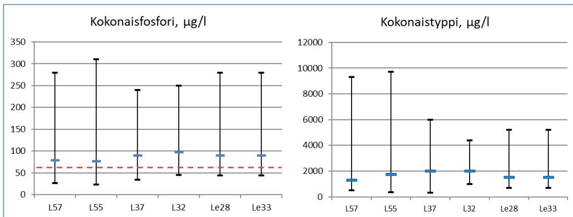
Kuva 4.37. Ravinnepitoisuuksien mediaanit, minimi- ja maksimiarvot Klaukkalan puhdistamon vaikutusalueella (L32 ja Le28) sekä vertailualueilla (L37 ja Le33) vuosina 2017-2019. Punainen katkoviiva kokonaisfosforikuvaajassa kuvaa hyvän tilan laatutavoitetta.
