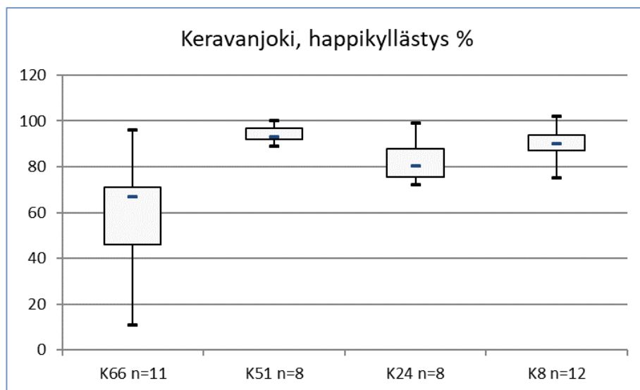
Kuva 6.8. Hapenkyllästysaste Ridasjärvessä kesällä (n=3) ja Keravanjoessa touko-syyskuussa (n=5) 2018. Arvot ovat havaintopaikan alin, ylin ja mediaani.
