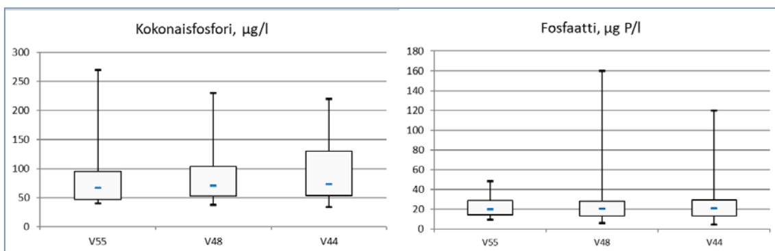
Kuva 4.32. Fosforipitoisuudet Vantaanjoen keskijuoksulla vuosina 2017-2019. Kuvan laatikkokaaviossa laatikon alareuna vastaa alaneljännestä, yläreuna yläneljännestä, alin ja ylin poikkiviiva ovat aineiston pienin ja suurin arvo, ja laatikossa oleva poikkiviiva on mediaani.
